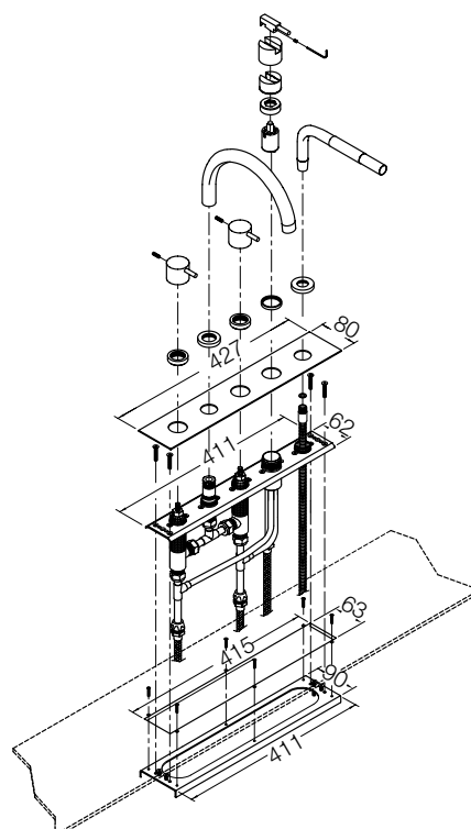
Til montage direkte på badekarkant (BK-B system)
