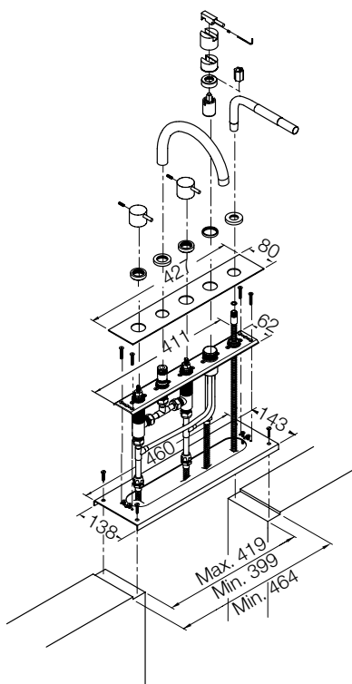
Uden montereramme og boks (BK-A system)
